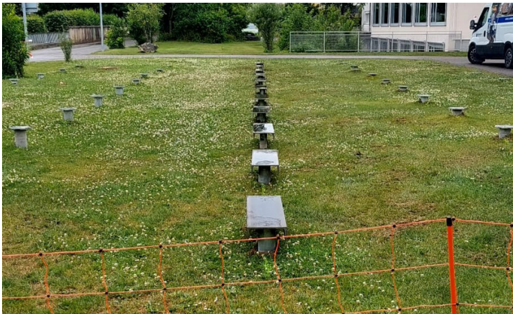
Zwischentraversen für stirnseitiges Doppelaufleger
